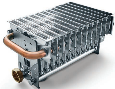
Queimador LowNOx com sistema de arrefecimento incorporado
